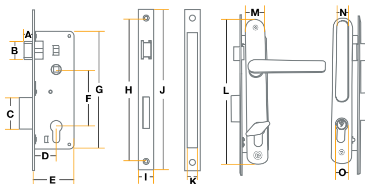
Medidas en mm
